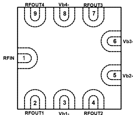
俯视透视图
